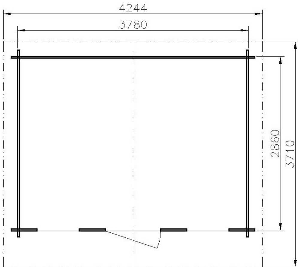
PŮDORYS
