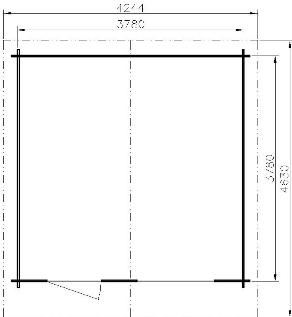
PŮDORYS
