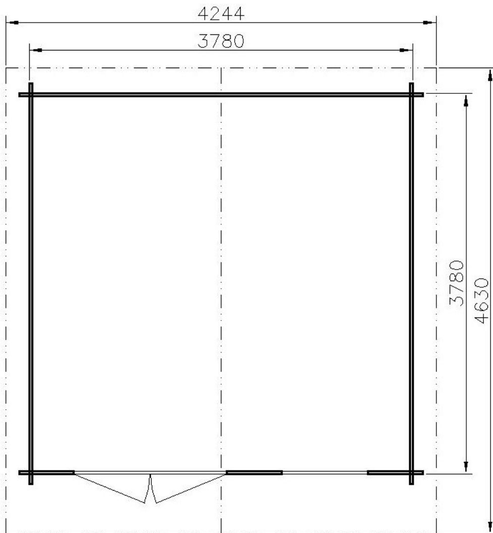
PŮDORYS
