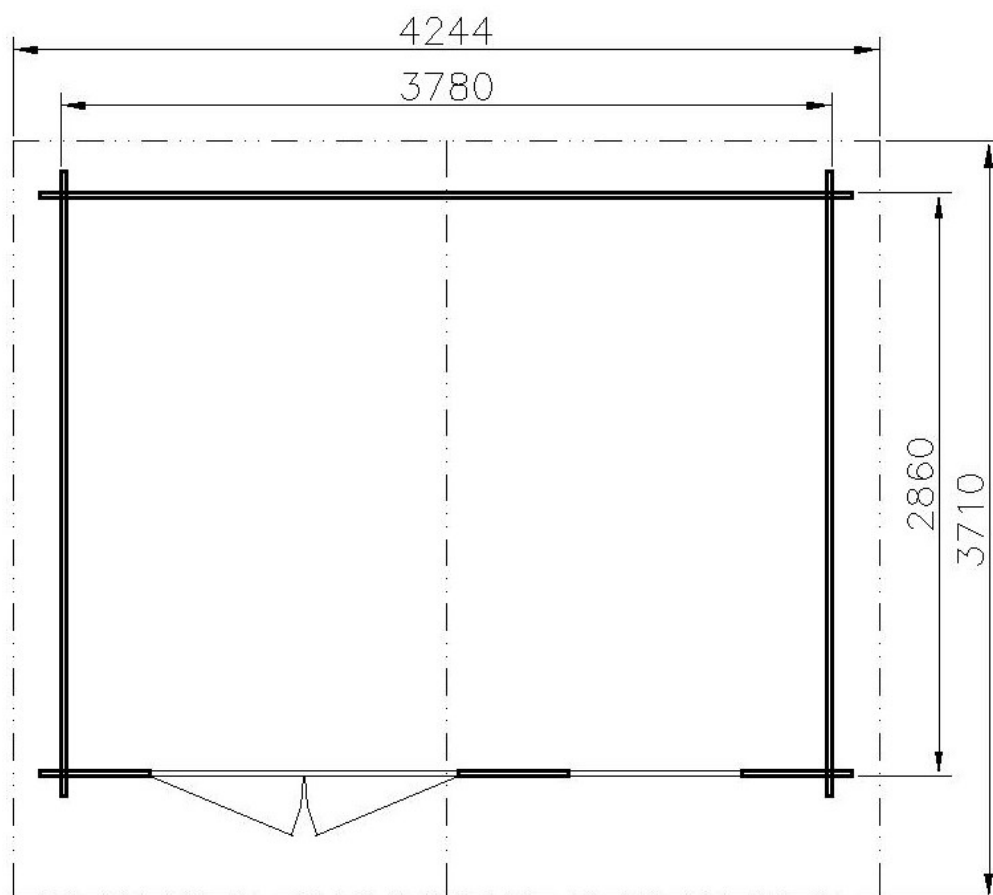
PŮDORYS
