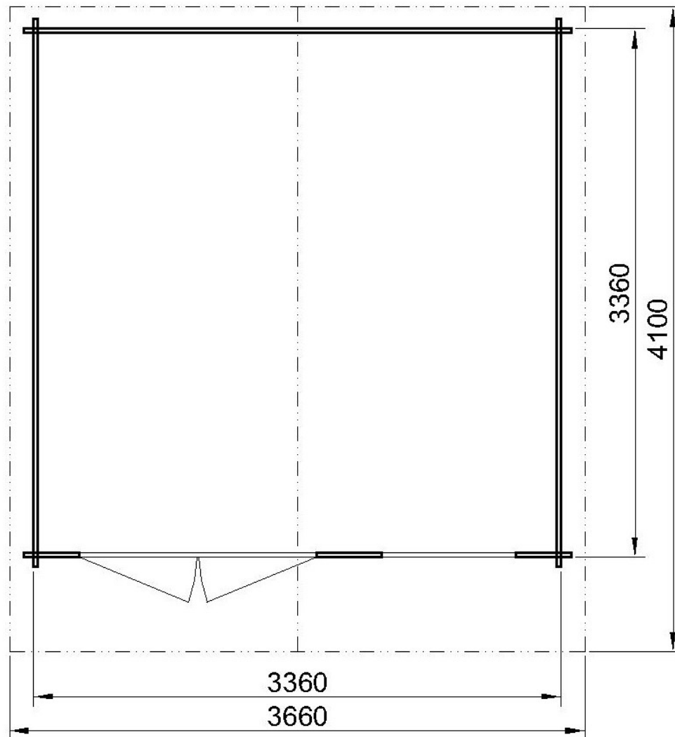
PŮDORYS
