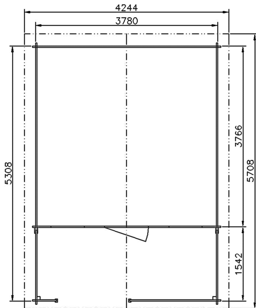
PŮDORYS
