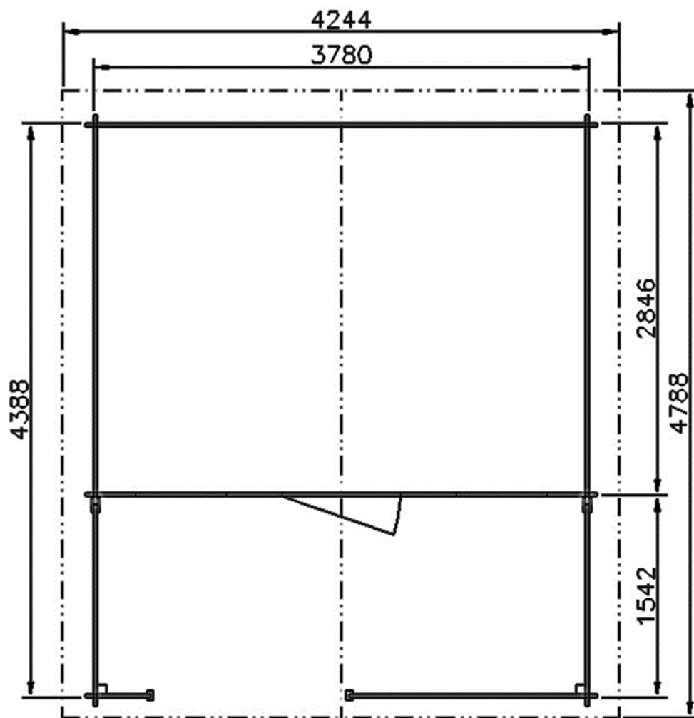
PŮDORYS
