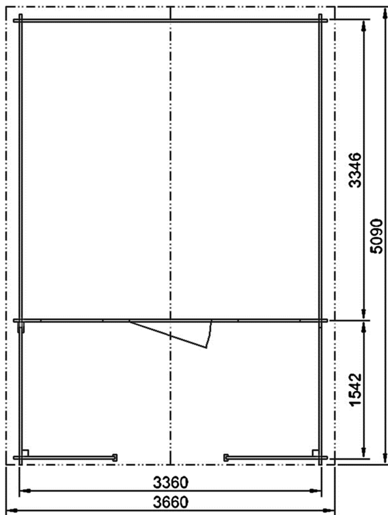
PŮDORYS
