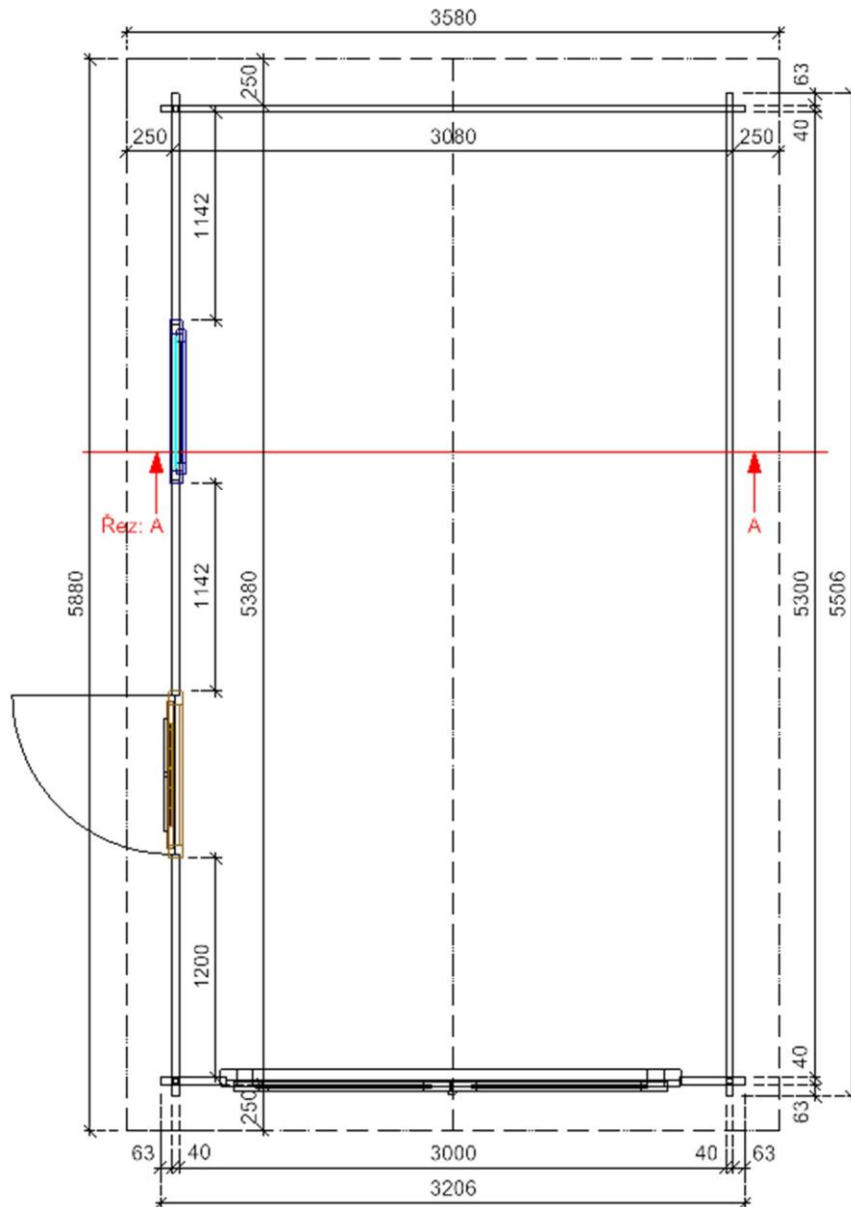
PÔDORYS
