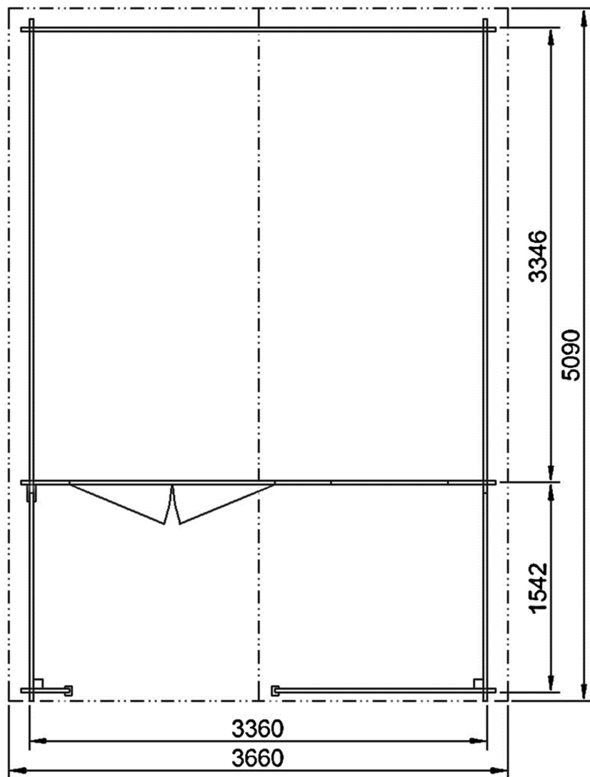
PŮDORYS
